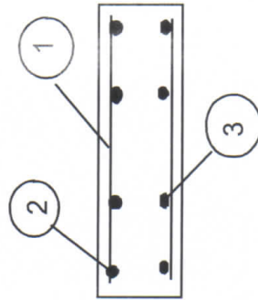
DETALIU ARMATURA CAPAC RIGOLA SC. 1:10 SECTIUNEA A-A
